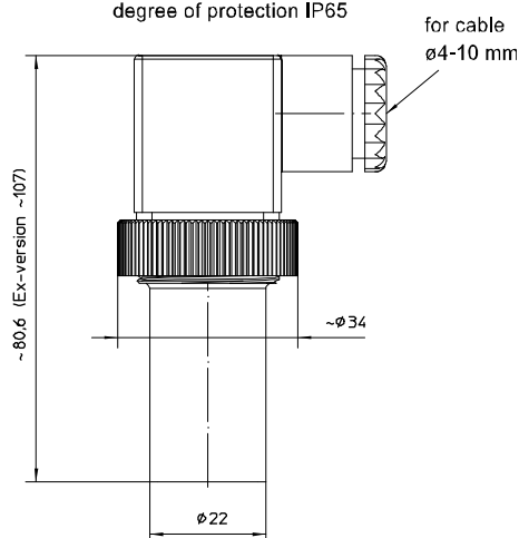
right-angle plug per DIN EN 175301-803-A degree of protection IP65
