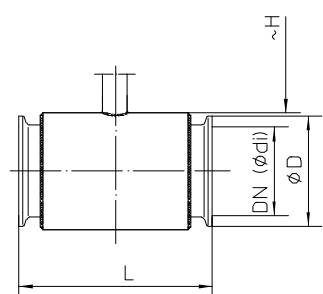
Clamp connection per ISO 2852, DIN 32676 or DIN 11864-3
