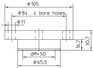
DRD-connection DN50 PN40 *
